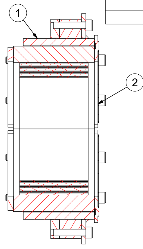
A-A ( 1 : 2 )
