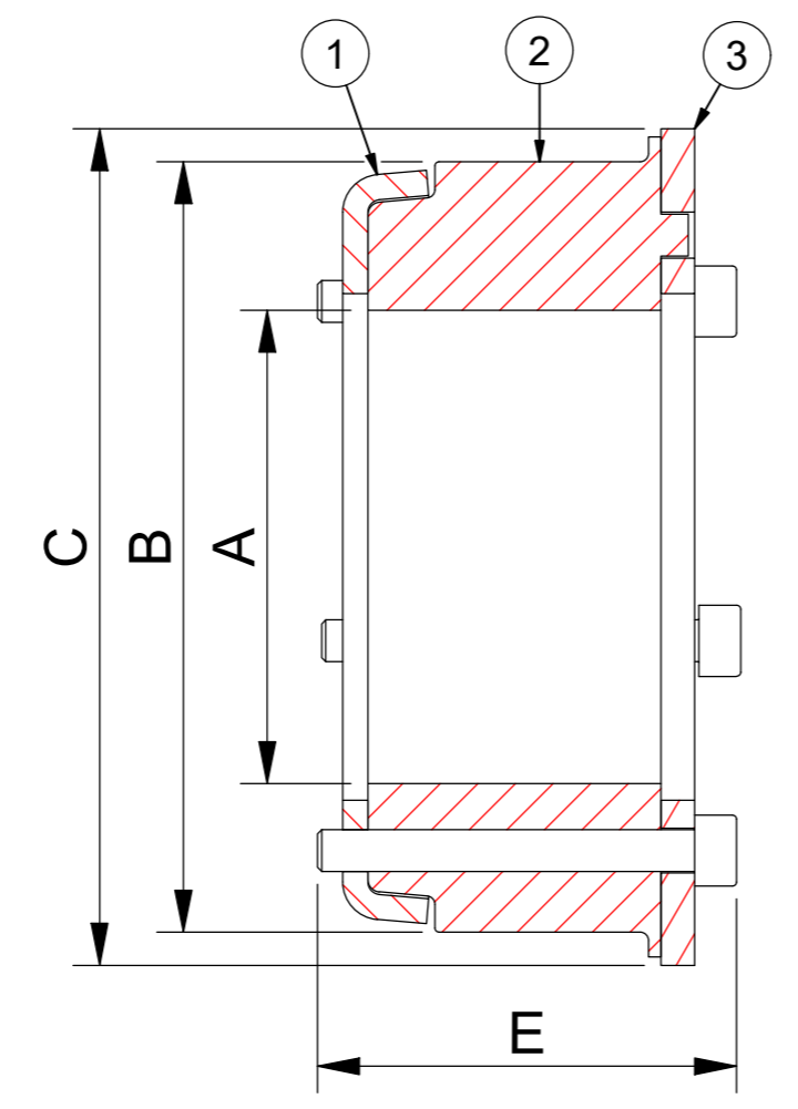
A-A (1:1)
